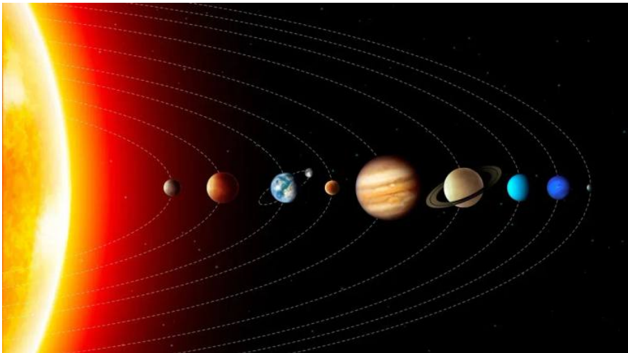
Sistema Solar mostrando el Sol y los ocho planetas en sus órbitas alrededor de la estrella
