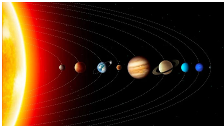
Sistema Solar mostrando el Sol y los ocho planetas en sus órbitas alrededor de la estrella
