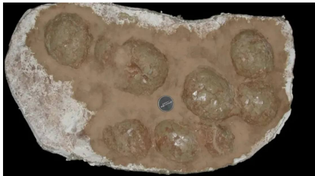
Fósiles de huevos de titanosaurios descubiertos en la Patagonia argentina, con escala de 1 cm
